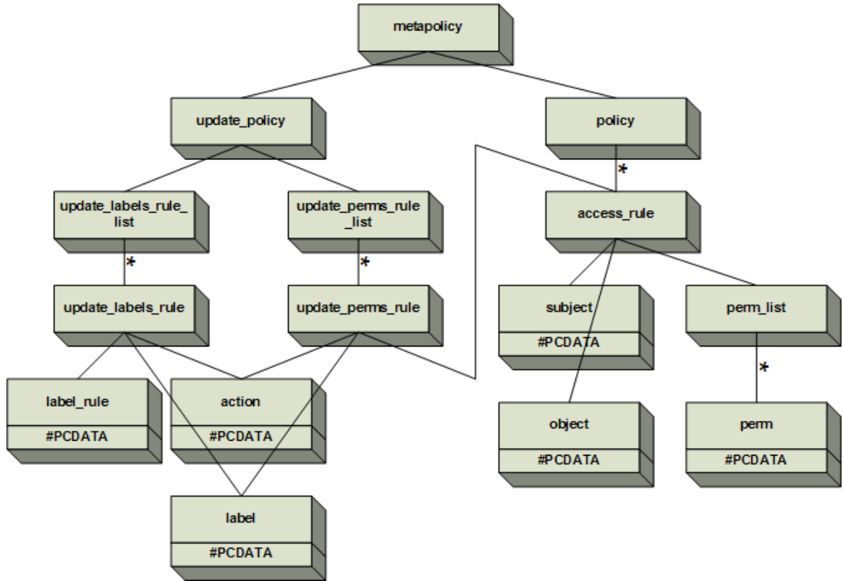
FIG. 7.7 – DTD pour la méta-politique \mathcal{MP}_{AC} .
