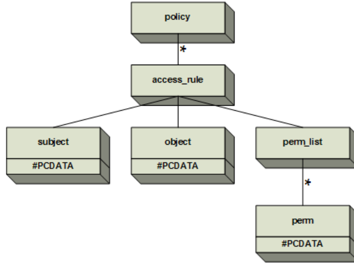
FIG. 7.6 – DTD pour la politique locale \mathcal{LR}_{AC}
