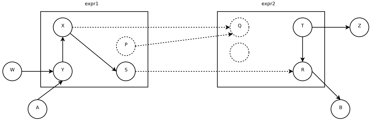
FIG. 6.5 – Regroupement des nœuds correspondant aux règles de la politique de modification. \mathcal{MR}_{\mathcal{AC}} du listing 6.2
