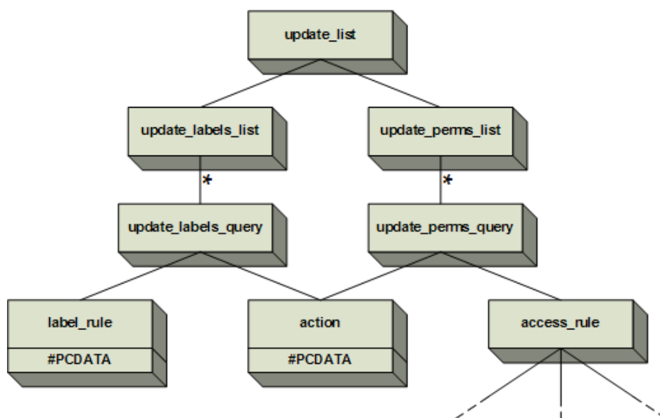
FIG. 7.8 – Requête de mise à jour en XML.
