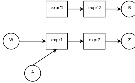
FIG. 6.12 – Graphe contracté global.
